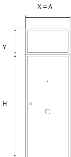
Altillo sencillo
