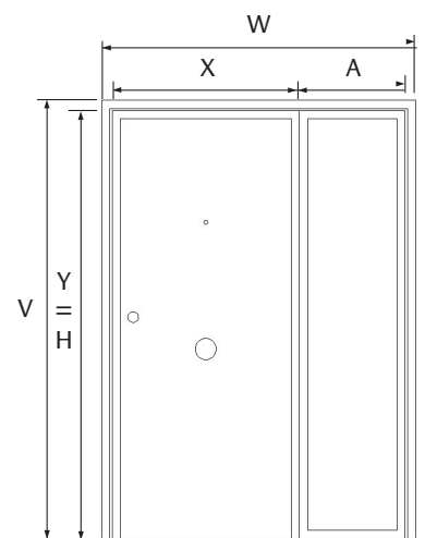
Fijos lateral en lado derecho
